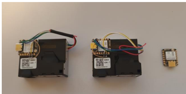
Фиг. 2. Система за изследване на въздуха използваща безжична комуникация базирана на протокола Thread
