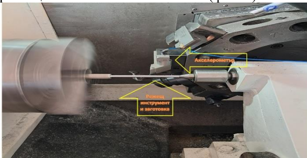
Фиг. 1. Измервателна установка.
