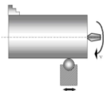
Фиг. 1. Схема на диамантено заглаждане (DB)
