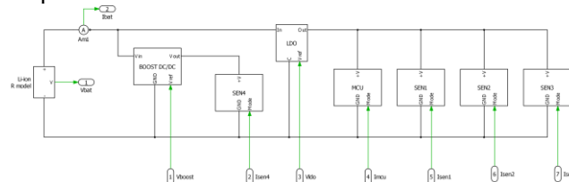
Фиг. 1. Системен модел на система за оценка на качеството на въздуха, разработен в средата на софтуерния продукт PLECS
