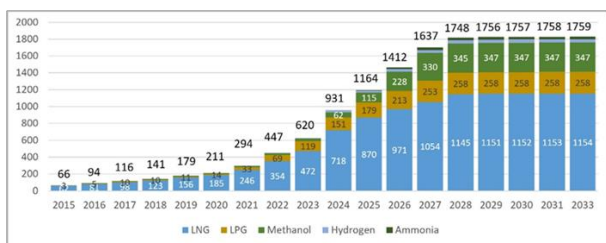
Фиг. 2. Изменение на броя на корабите използващи алтернативни горива (VERACITY by DNV)
