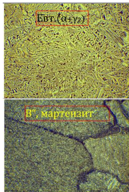
Фиг. 4. Микроструктура в зоната на залятия бронз, а/ проба 1 залята структура, б/ проба 2 залята и закалена от 920°C
