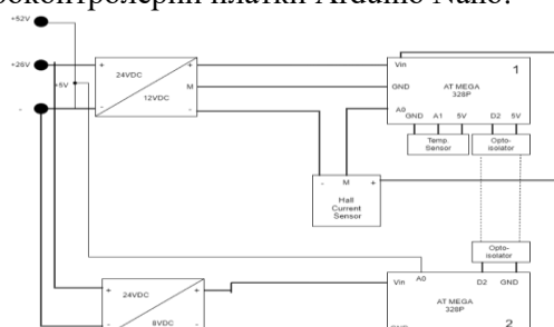
Фигура 2. Блок-схема на изработения даталогер
