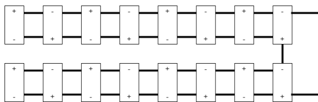
Фигура 1. Схема на свързване на клетките
