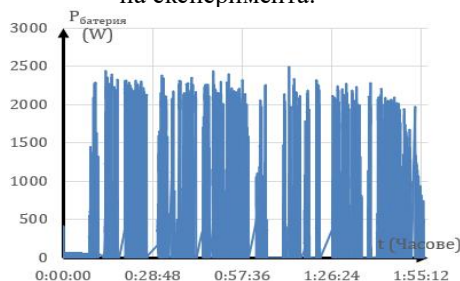
Фиг. 4. Консумирана мощност от електродвигателя по време на експеримента.
