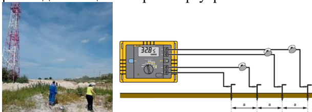
Фиг. 1. Полеви измервания по метода Венер- \alpha
